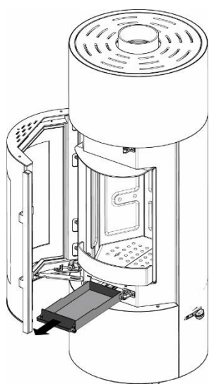
Rysunek 11. Czyszczenie ogrzewacza
