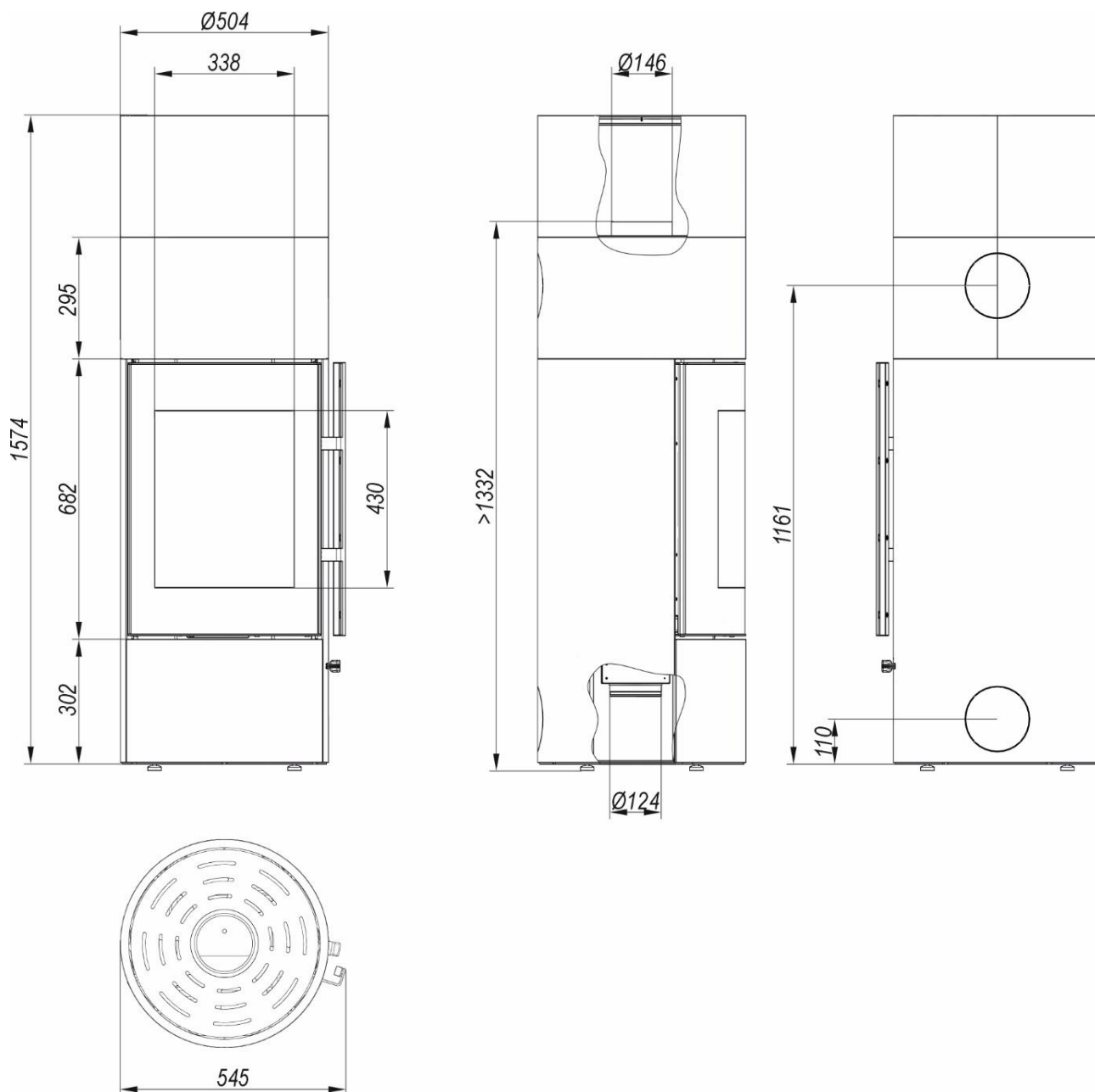
Rysunek 3. Wymiary (mm) ogrzewacza pokojowego DEFRO HOME ORION PLS 2.0
