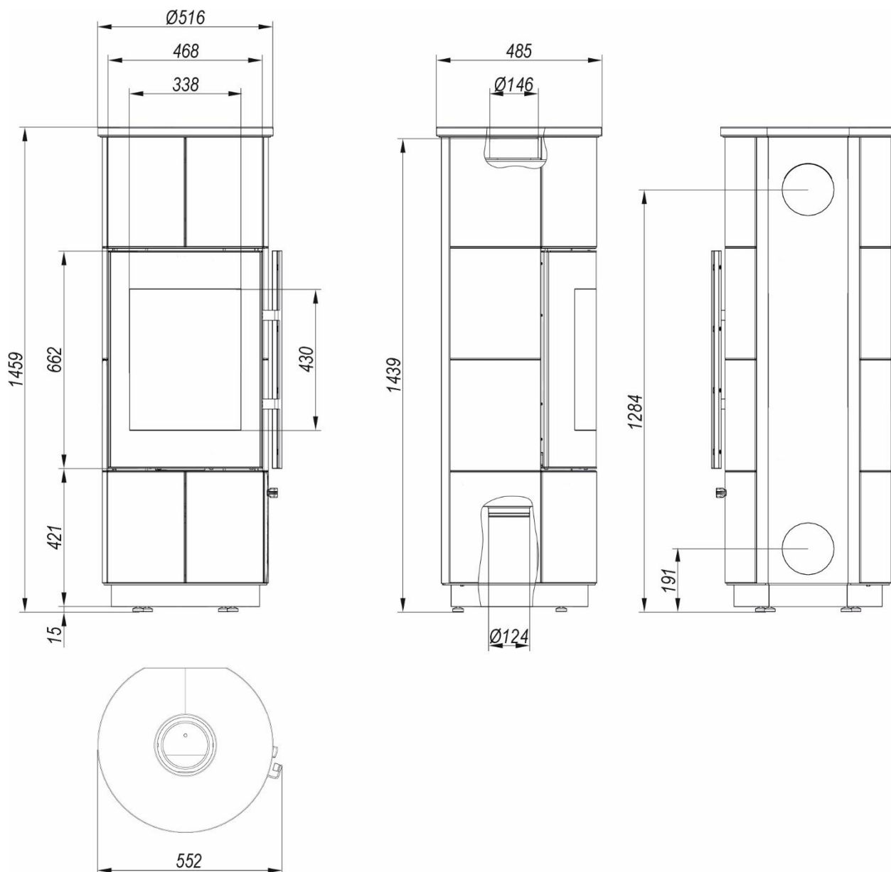
Rysunek 4. Wymiary (mm) ogrzewacza pokojowego DEFRO HOME ORION KRM 2.0
