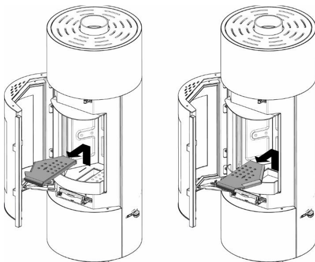
Krok 1. Wyjąć obie części rusztu.
