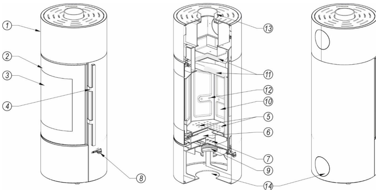
Rysunek 1. Budowa ogrzewacza serii DEFRO HOME ORION 2.0
