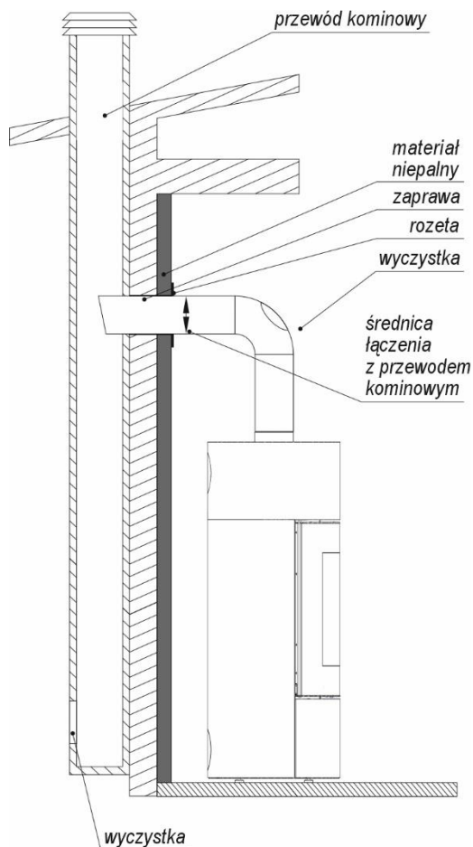
Rysunek 8. Podłączenie ogrzewacza serii DEFRO HOME ORION 2.0 do przewodu kominowego.
