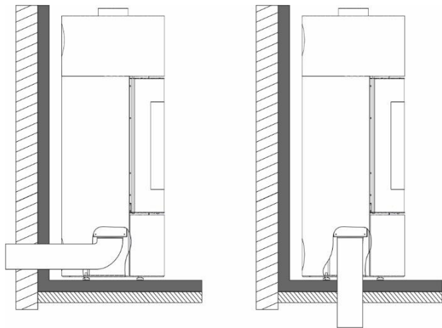
Rysunek 7. Podłączenie ogrzewacza serii DEFRO HOME ORION 2.0 do zewnętrznego wlotu powietrza
