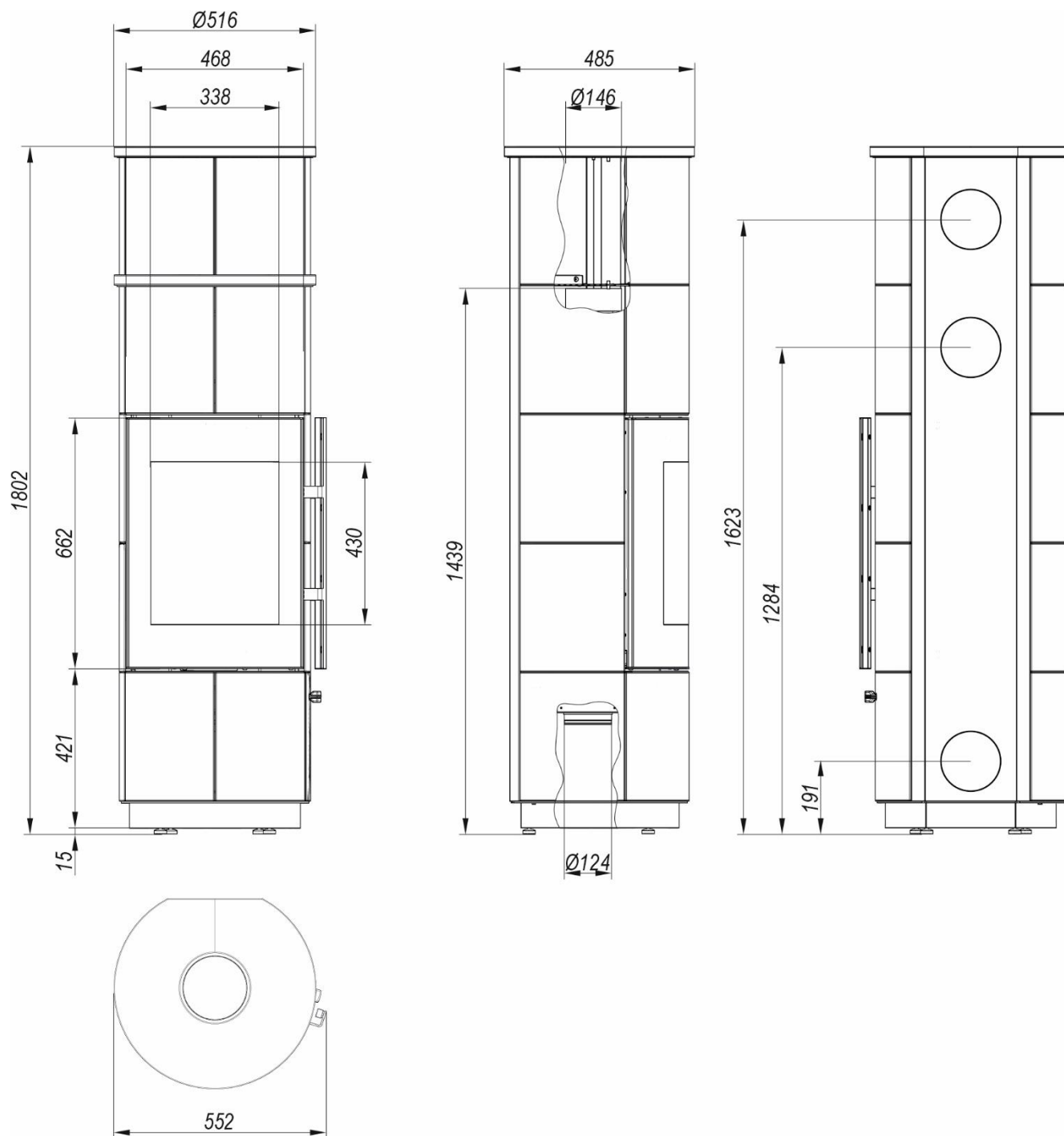
Rysunek 5. Wymiary (mm) ogrzewacza pokojowego DEFRO HOME ORION KRM PLS 2.0
