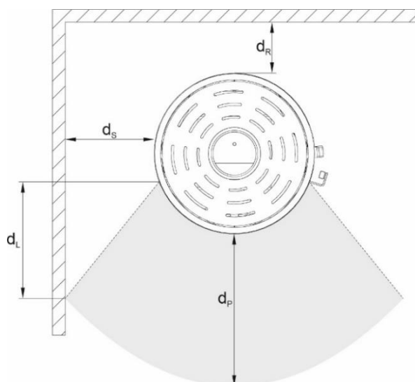
Rysunek 6. Ustawienia ogrzewacza - odległości do materiałów palnych
