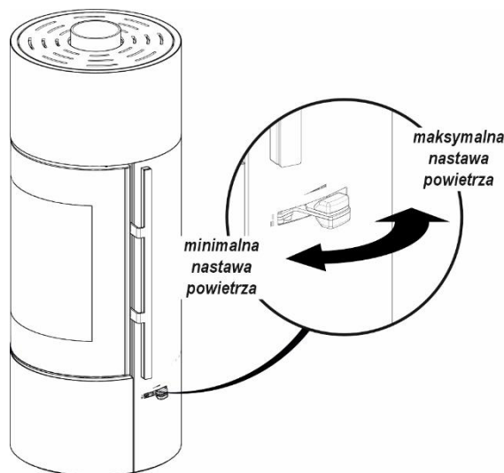
Rysunek 9. Regulacja dopływu powietrza
