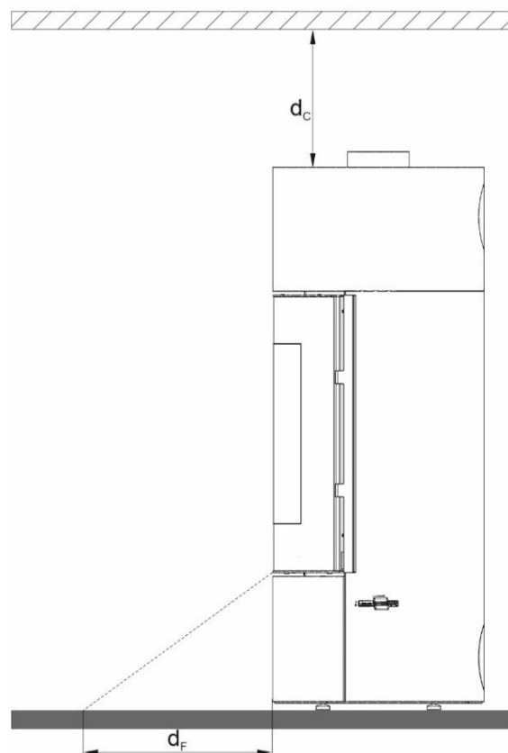
Rysunek 6. Ustawienia ogrzewacza - odległości do materiałów palnych
