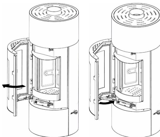
Rysunek 12. Mechanizm blokady drzwi
