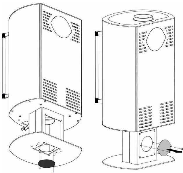
Rysunek 13. Podłączenie ogrzewacza serii TOP
