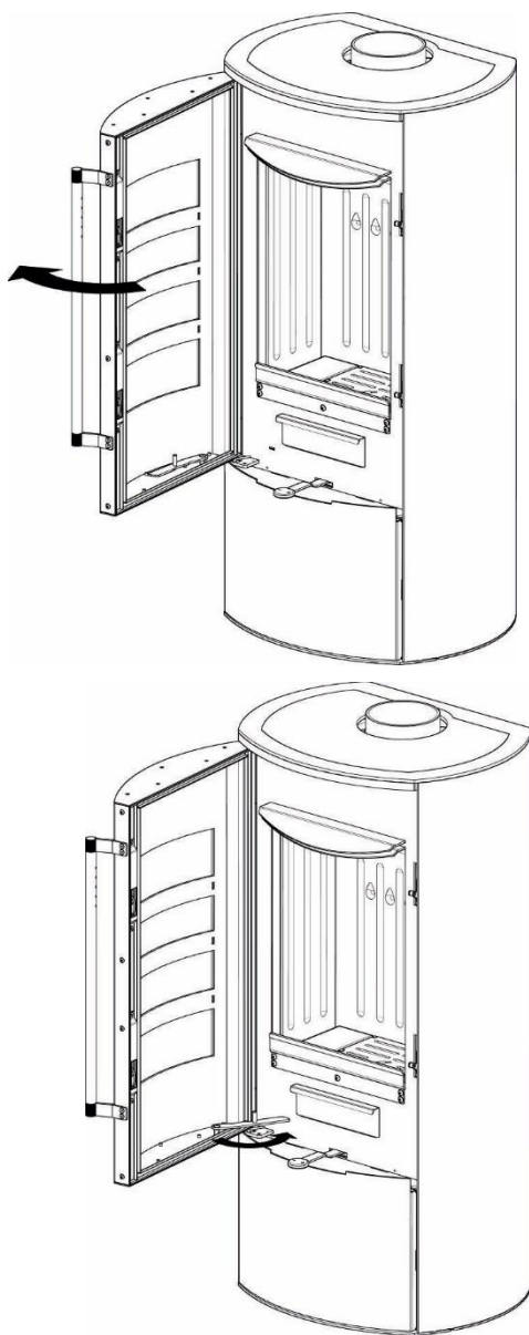
Rysunek 19. Mechanizm blokady drzwi
