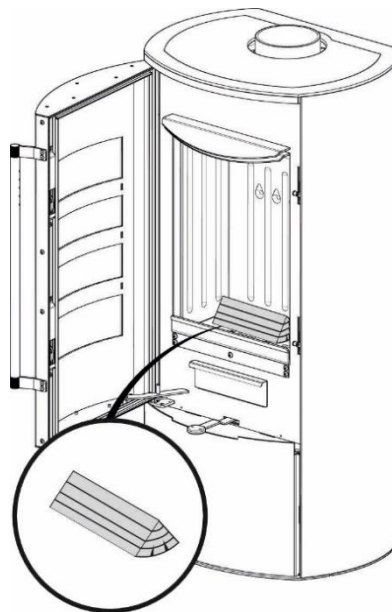
Rysunek 17. Sposób ułożenia paliwa
