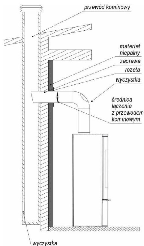
Rysunek 14. Możliwości podłączenie ogrzewacza do przewodu kominowego.
