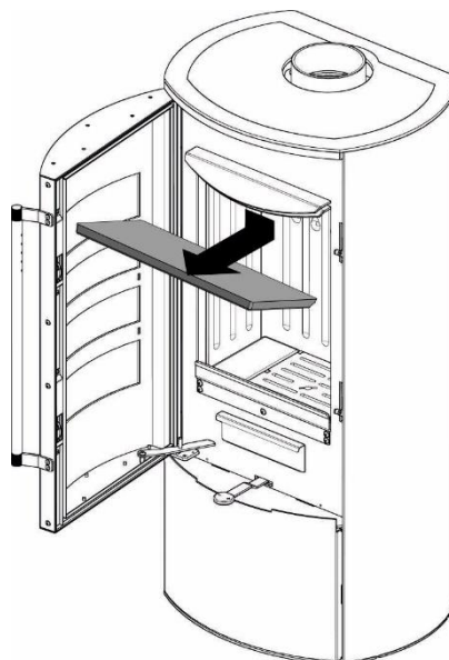
Krok 1. Jako pierwszy element należy zdemontować deflektor.
