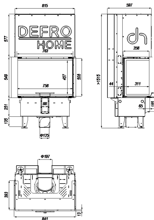
Rysunek 31. Wymiary wkładu kominkowego DEFRO HOME INTRA SM C G
