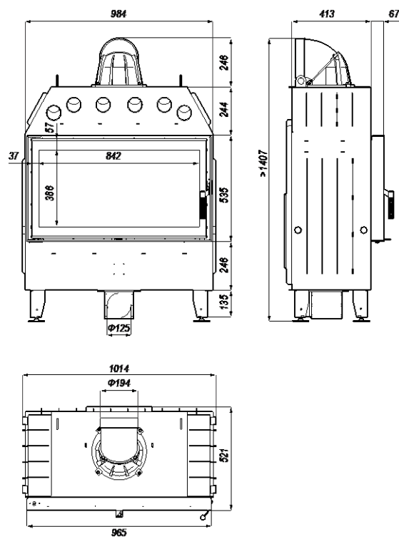
Rysunek 7. Wymiary wkładu kominkowego DEFRO HOME INTRA LA.
