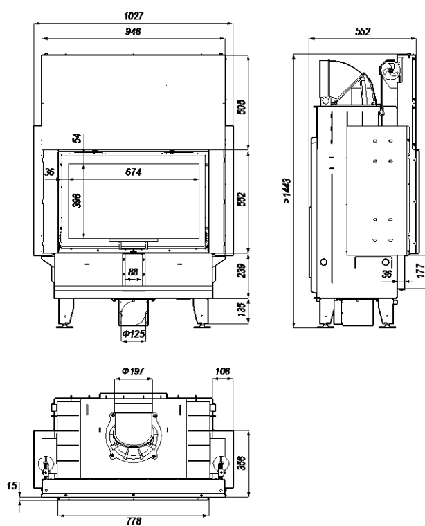
Rysunek 13. Wymiary wkładu kominkowego DEFRO HOME INTRA ME G.
