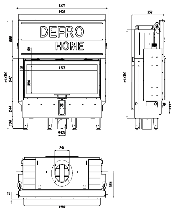
Rysunek 15. Wymiary wkładu kominkowego DEFRO HOME INTRA XLA G
