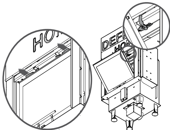
Rysunek 41. Umieszczenie rygli pozwalających na otwarcie drzwi gilotynowych w pozycji uchylnej wkładu kominkowego DEFRO HOME INTRA w wersji G.
