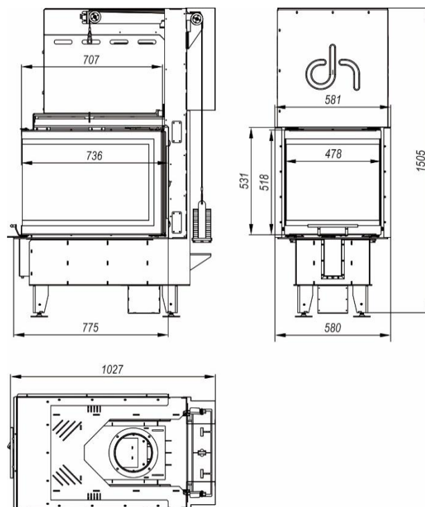
Rysunek 33. Wymiary wkładu kominkowego DEFRO HOME INTRA SM U G
