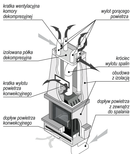
Rysunek 35. System dystrybucji gorącego powietrza.
