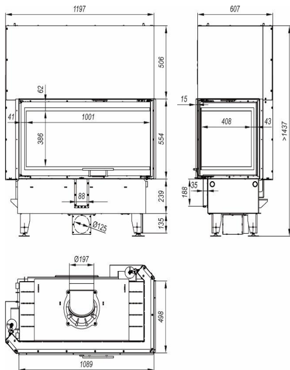
Rysunek 18. Wymiary wkładu kominkowego DEFRO HOME INTRA LA BP G
