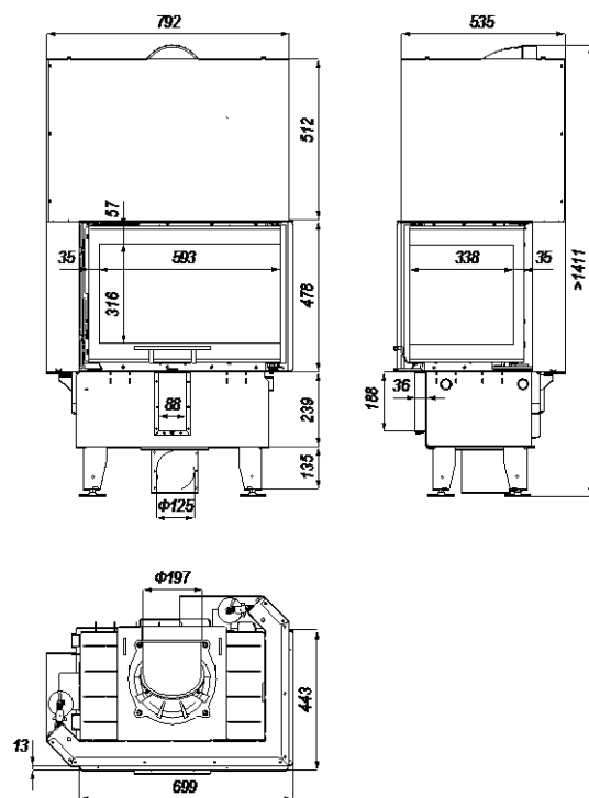
Rysunek 20. Wymiary wkładu kominkowego DEFRO HOME INTRA SM BP MINI G.
