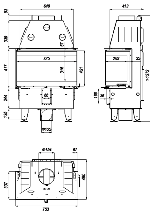
Rysunek 29. Wymiary wkładu kominkowego DEFRO HOME INTRA SM C.
