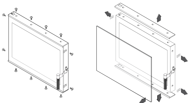
Rysunek 44. Demontaż szyby w drzwiach.
