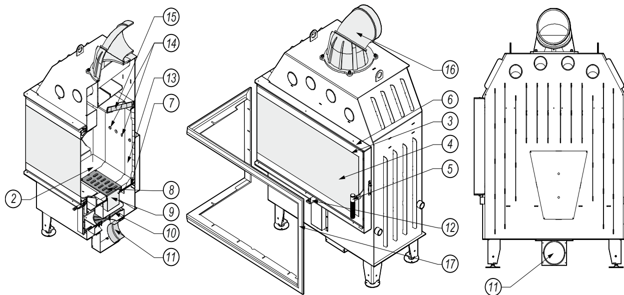
Rysunek 3. Budowa wkładu kominkowego DEFRO HOME INTRA BL i BP(odbicie lustrzane wersji BL) z drzwiami rozwieralnymi i szybą boczną.
