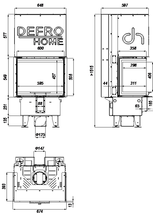
Rysunek 30. Wymiary wkładu kominkowego DEFRO HOME INTRA XSM C G
