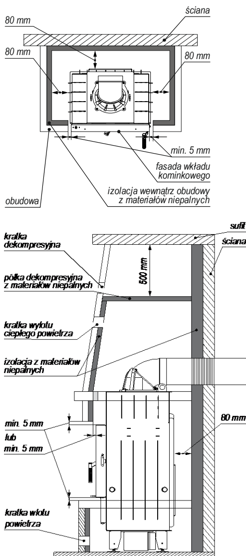
Rysunek 34. Przykładowa zabudowa wkładu kominkowego.
