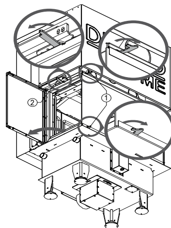
Rysunek 43. Umieszczenie rygli pozwalających na otwarcie szyb bocznych w drzwiach podnoszonych w wersji C wkładu kominkowego DEFRO HOME INTRA C G.
