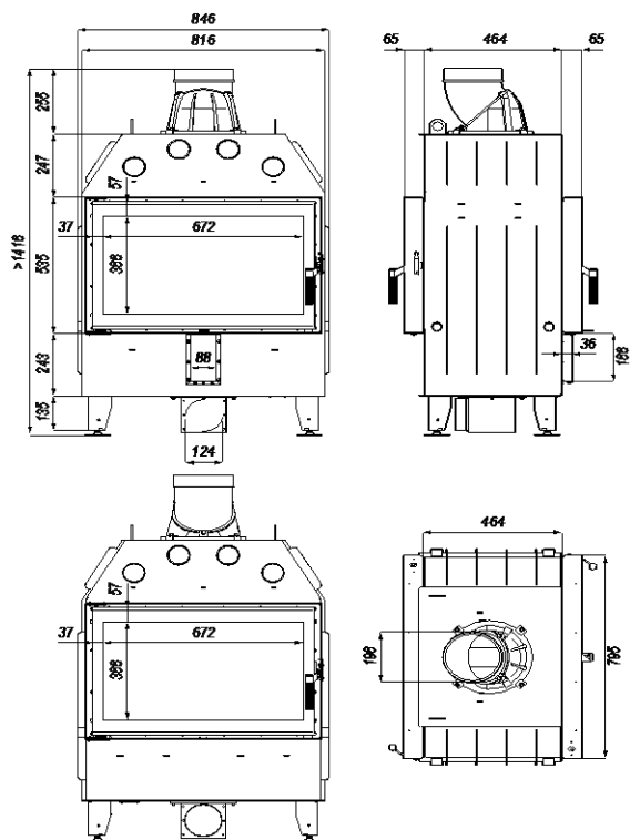
Rysunek 22. Wymiary wkładu kominkowego DEFRO HOME INTRA ME T.
