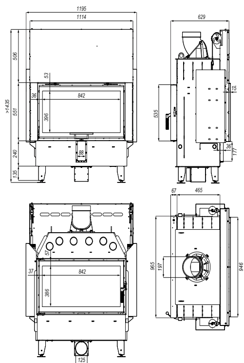
Rysunek 26. Wymiary wkładu kominkowego DEFRO HOME INTRA LA T G.
