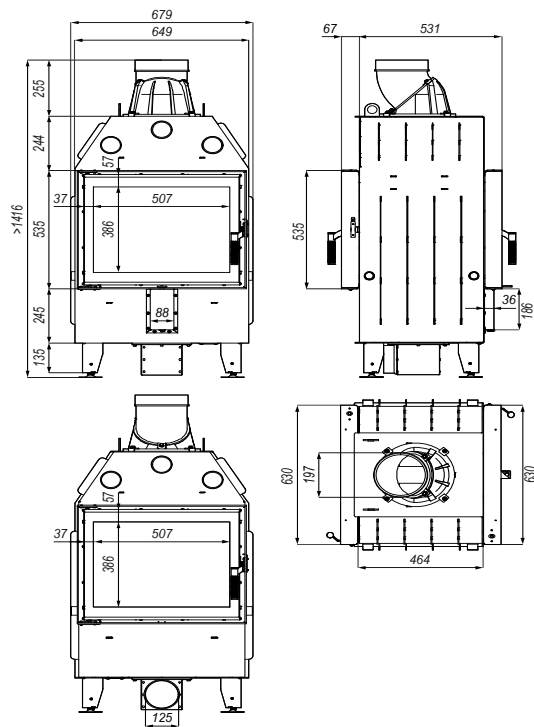
Rysunek 21. Wymiary wkładu kominkowego DEFRO HOME INTRA SM T.
