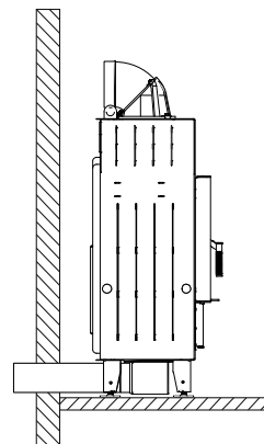
Rysunek 36. Podłączenie wkładu kominkowego do zewnętrznego wlotu powietrza.
