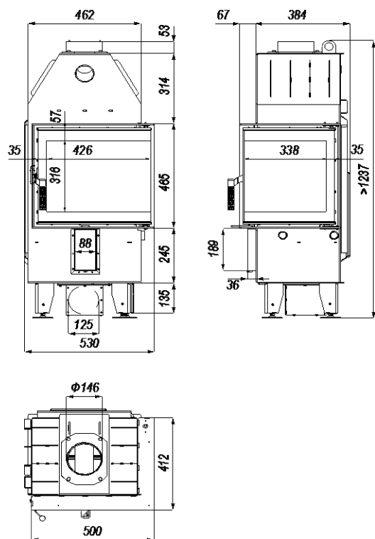
Rysunek 10. Wymiary wkładu kominkowego DEFRO HOME INTRA XSM BP MINI
