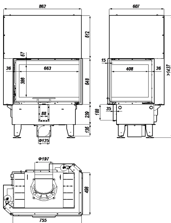
Rysunek 16. Wymiary wkładu kominkowego DEFRO HOME INTRA SM BP G.
