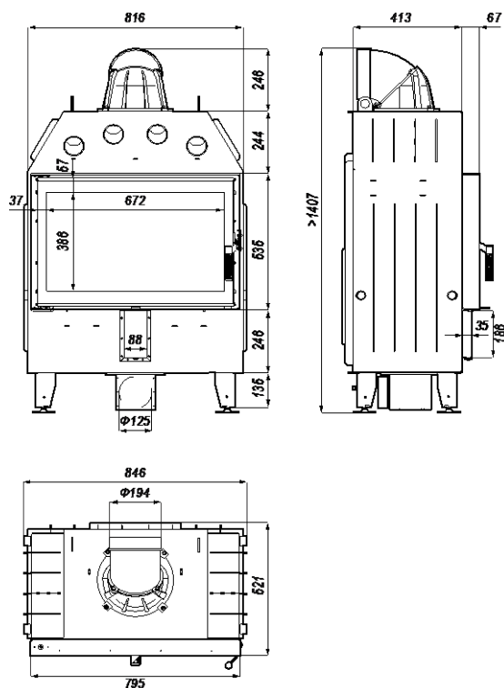
Rysunek 6. Wymiary wkładu kominkowego DEFRO HOME INTRA ME
