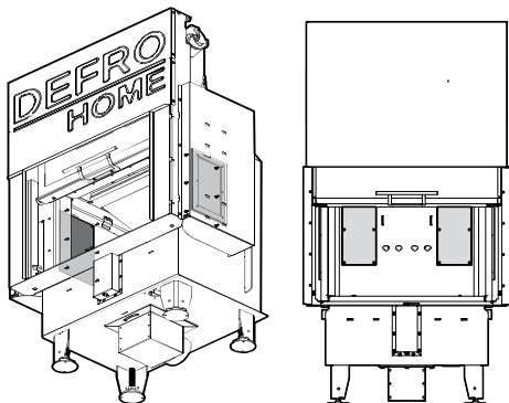
Rysunek 45. Umieszczenie pokryw otworów rewizyjnych we wkładach: DEFRO HOME INTRA wersji G (po lewej) i DEFRO HOME INTRA wersji C G (po prawej).
