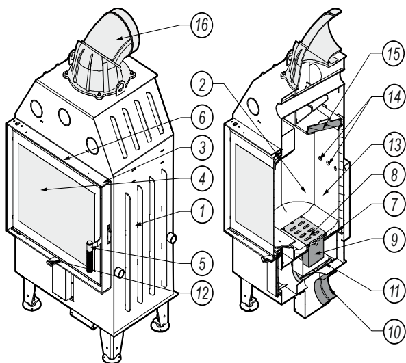
Rysunek 1. Budowa wkładu kominkowego DEFRO HOME INTRA z drzwiami rozwieralnymi.
