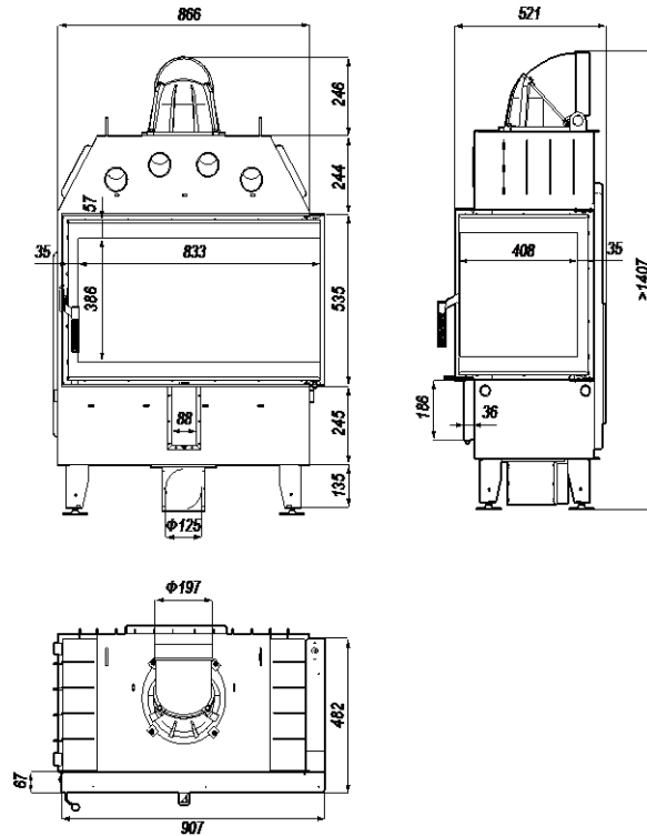
Rysunek 9. Wymiary wkładu kominkowego DEFRO HOME INTRA ME BP.
