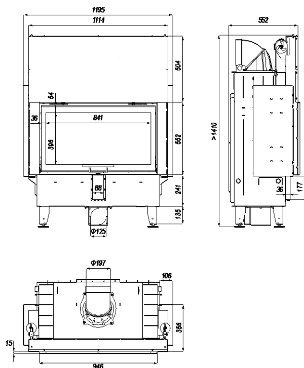
Rysunek 14. Wymiary wkładu kominkowego DEFRO HOME INTRA LA G
