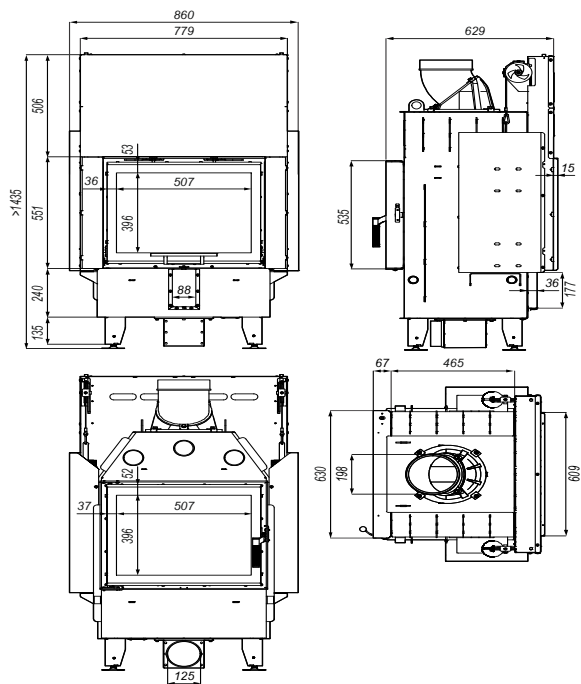
Rysunek 24. Wymiary wkładu kominkowego DEFRO HOME INTRA SM T G
