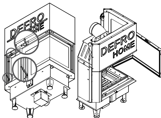
Rysunek 42. Umieszczenie rygli pozwalających na otwarcie drzwi w pozycji uchylnej w drzwiach gilotynowych z szybą boczną kominka DEFRO HOME INTRA w wersji BP(BL) G.
