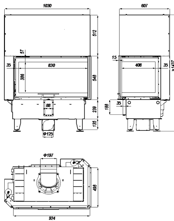
Rysunek 17. Wymiary wkładu kominkowego DEFRO HOME INTRA ME BP G.
