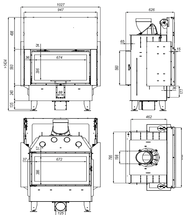
Rysunek 25. Wymiary wkładu kominkowego DEFRO HOME INTRA ME T G.
