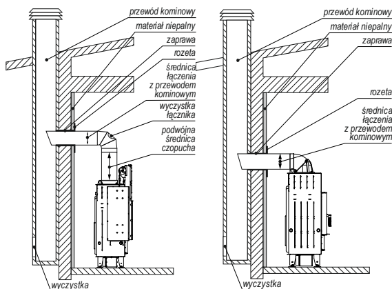
Rysunek 37. Podłączenie wkładu kominkowego do przewodu kominowego w zależności od wersji (po lewej wersji XSM i XLA, po prawej pozostałe).
