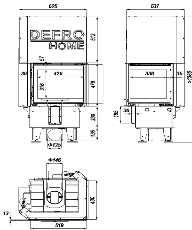
Rysunek 19. Wymiary wkładu kominkowego DEFRO HOME INTRA XSM BP MINI G.
