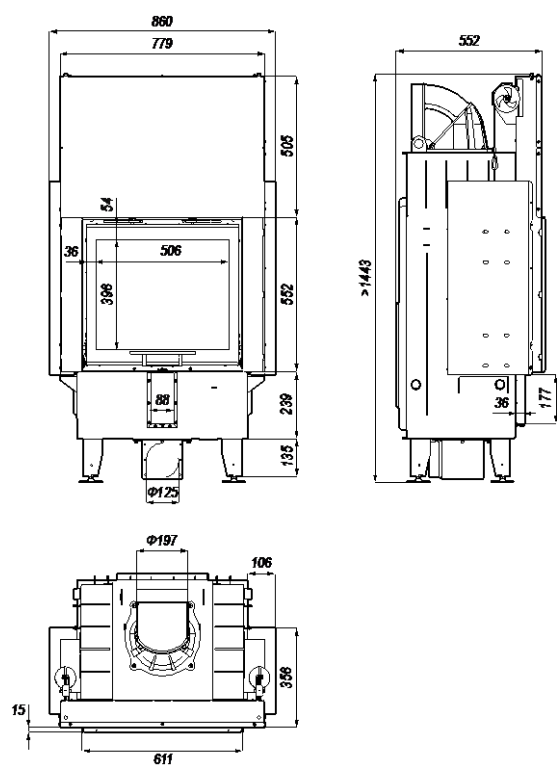
Rysunek 12. Wymiary wkładu kominkowego DEFRO HOME INTRA SM G
