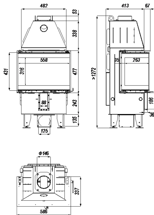
Rysunek 27. Wymiary wkładu kominkowego DEFRO HOME INTRA XSM C.
