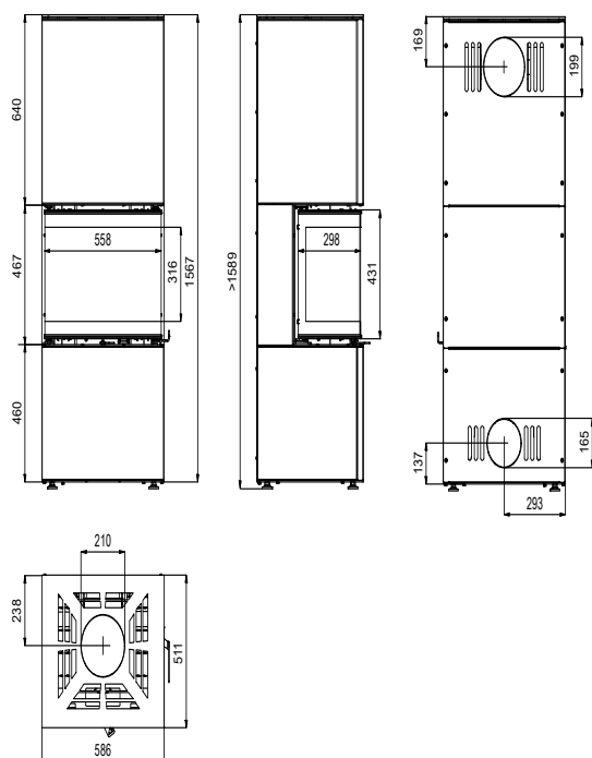
Rysunek 28. Wymiary wkładu kominkowego DEFRO HOME INTRA XSM C razem z zabudową w opcji COMPACT 1.
