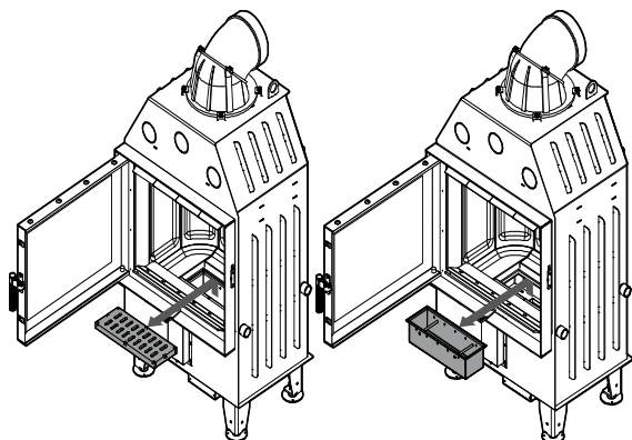
Rysunek 40. Wyjęcie rusztu i popielnika w celu jego opróżnienia.
