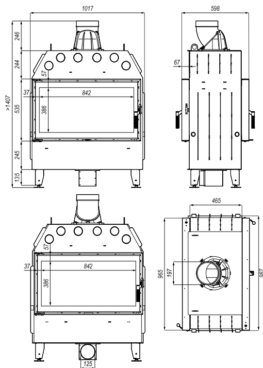
Rysunek 23. Wymiary wkładu kominkowego DEFRO HOME INTRA LA T
