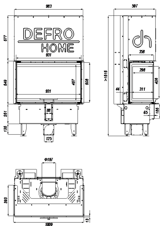
Rysunek 32. Wymiary wkładu kominkowego DEFRO HOME INTRA ME C G
