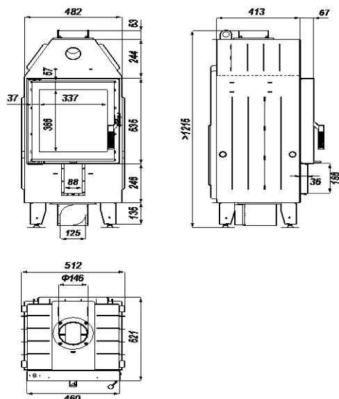
Rysunek 4. Wymiary wkładu kominkowego DEFRO HOME INTRA XSM
