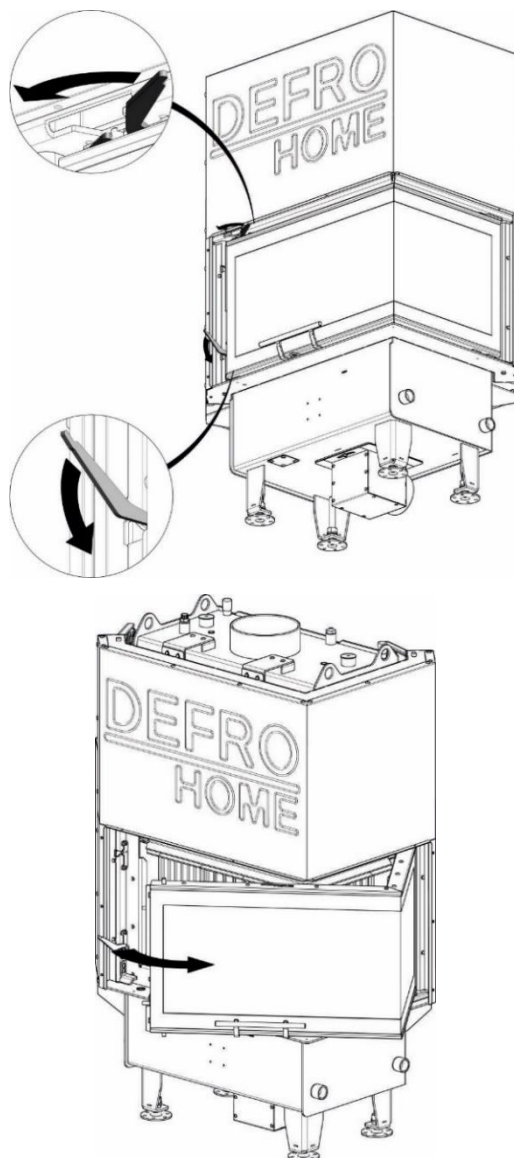
Rysunek 25. Umieszczenie rygla pozwalającego na otwarcie drzwi gilotynowych w pozycji rozwieralnej wkładu kominkowego DEFRO HOME RIVA BP SHORT w wersji G oraz widok drzwi w pozycji rozwieralnej. (BL G odbicie lustrzane).
