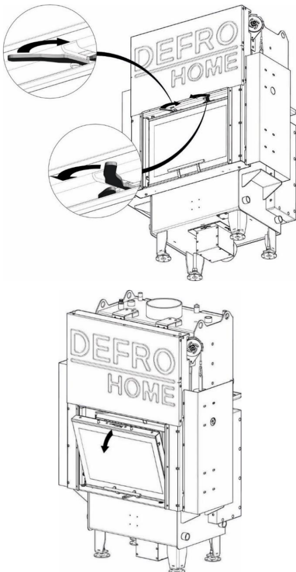
Rysunek 24. Umieszczenie rygla pozwalającego na otwarcie drzwi gilotynowych w pozycji uchylnej wkładu kominkowego DEFRO HOME RIVA SHORT w wersji G.
