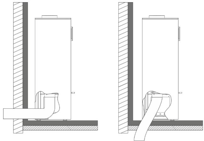
Rysunek 5. Podłączenie ogrzewacza pomieszczeń do zewnętrznego wlotu powietrza
