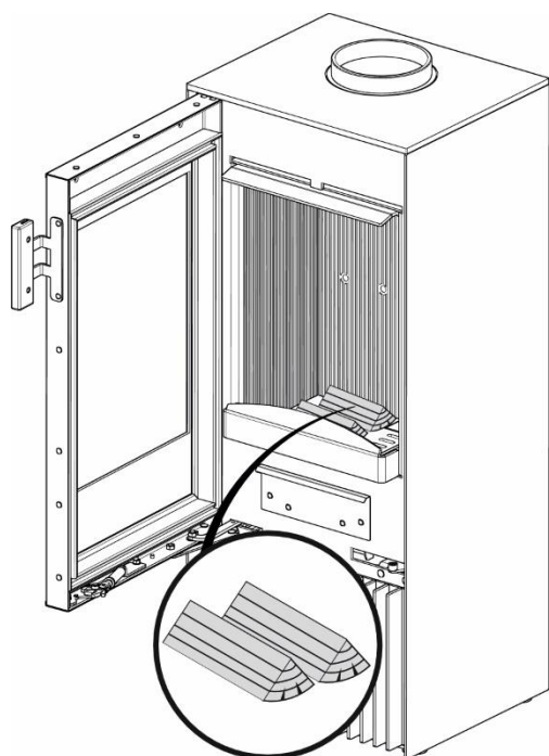
Rysunek 8. Sposób ułożenia paliwa.
