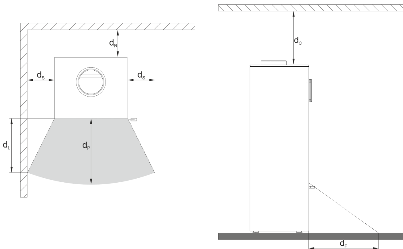
Rysunek 4. Odległości do materiałów palnych
