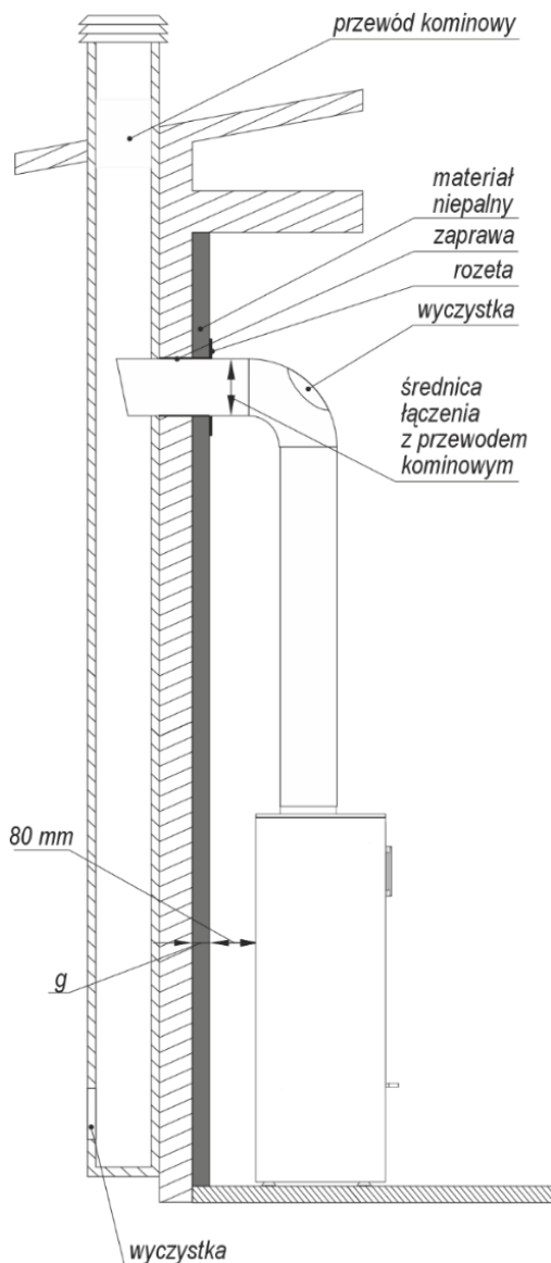
Rysunek 6. Podłączenie ogrzewacza pomieszczeń do przewodu kominowego.
