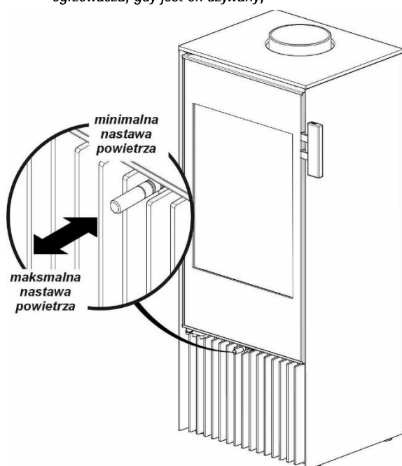
Rysunek 7. Ustawienie suwaka regulacji dopływu powietrza.
