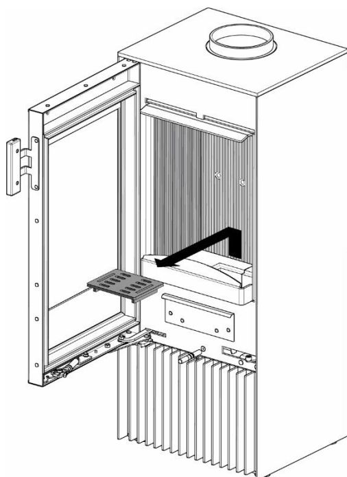
Rysunek 9. Ruszt
