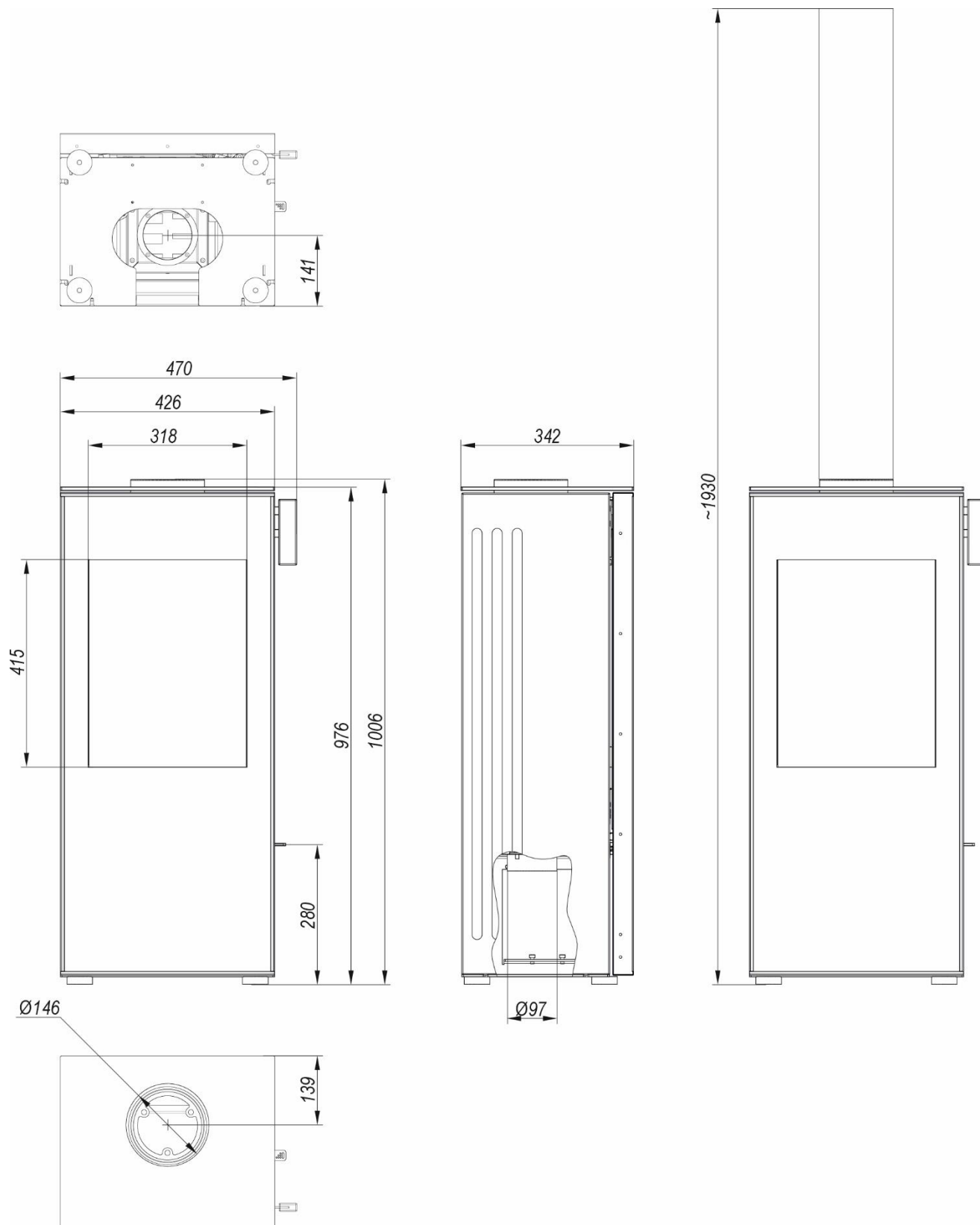
Rysunek 3. Wymiary ogrzewacza DEFRO HOME BRAS
