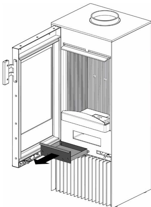
Rysunek 10. Szuflada na popiół
