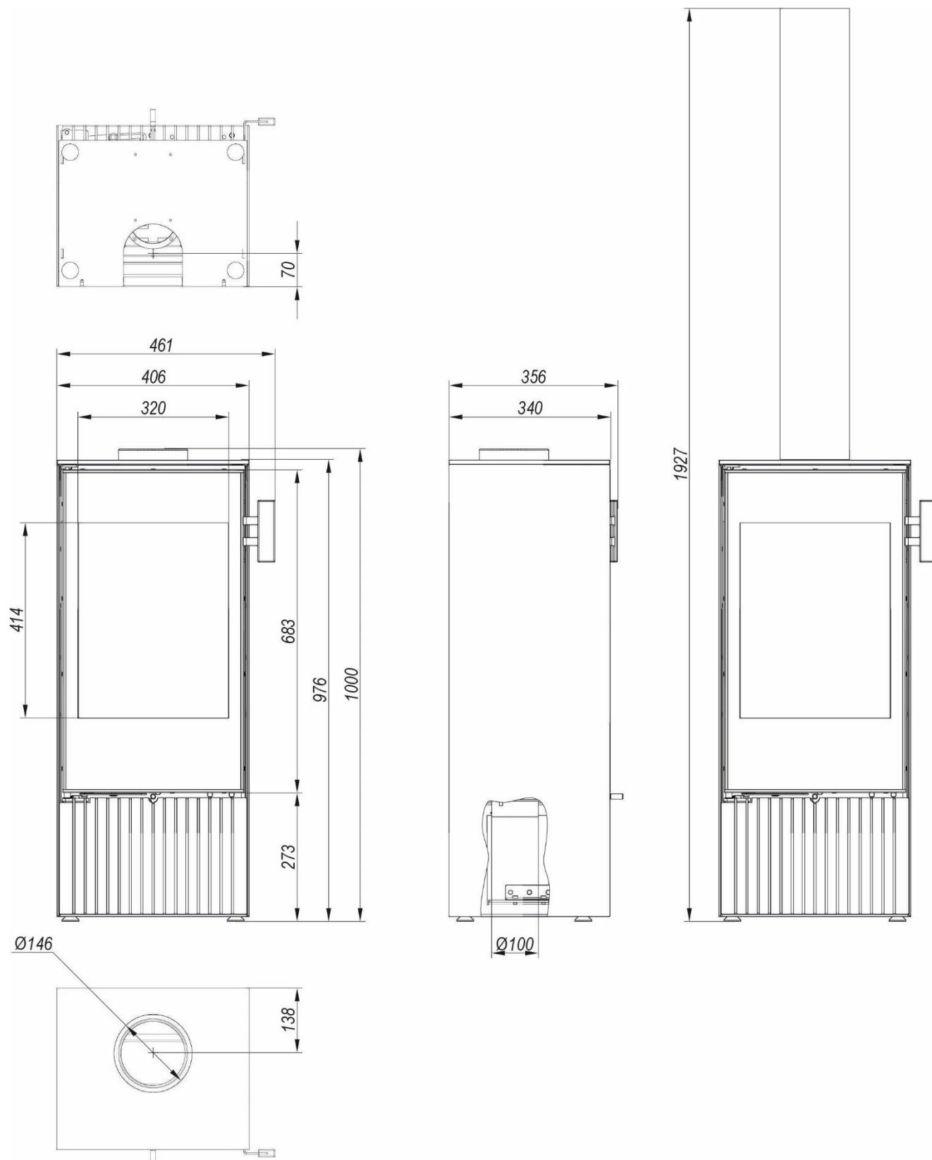
Rysunek 2. Wymiary ogrzewacza DEFRO HOME ADEO
