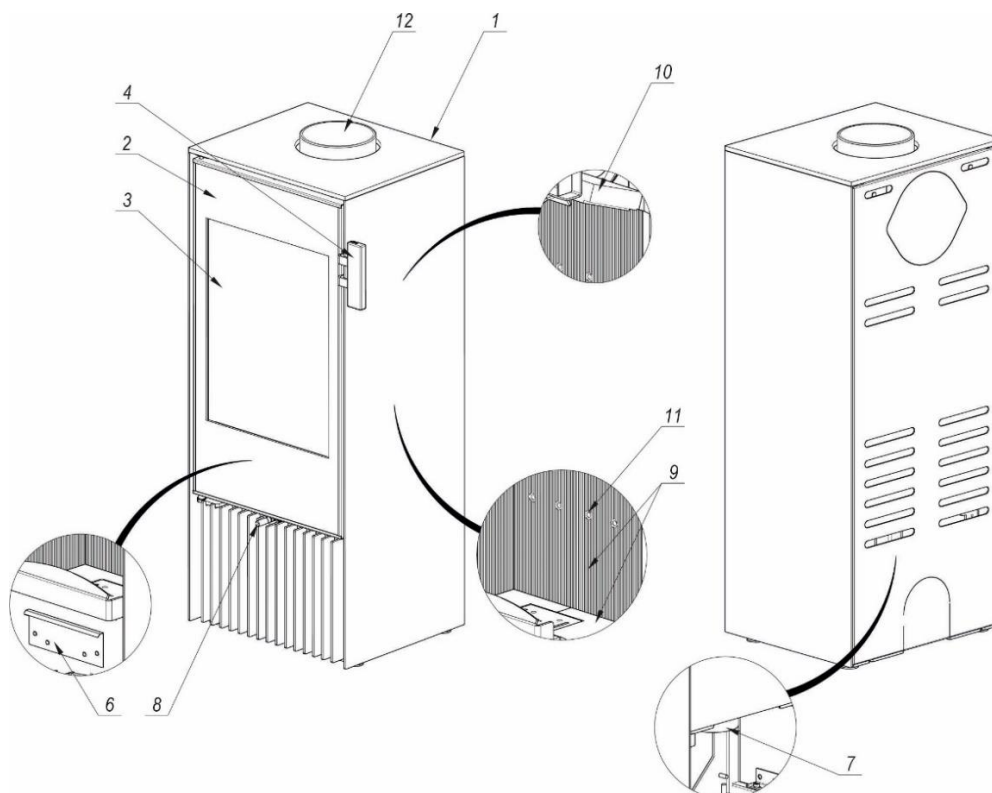
Rysunek 1. Budowa ogrzewacza pomieszczeń DEFRO HOME ADEO
