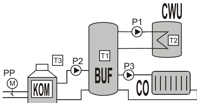
Rys.1a Podstawowy układ pracy regulatora
