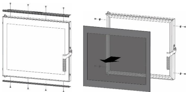
Rysunek 34. Demontaż szyby w drzwiach.
