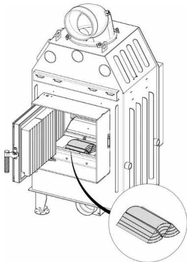
Rysunek 26 Sposób ułożenia paliwa dla wersji TZ
