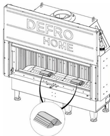
Rysunek 25 Sposób ułożenia paliwa dla wersji XL
