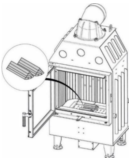
Rysunek 24 Sposób ułożenia paliwa
