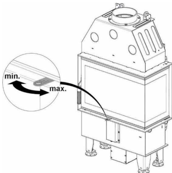
Rysunek 14. Ustawienie suwaka regulacji dopływu powietrza.
