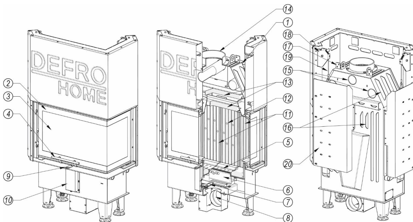
Rysunek 4. Budowa wkładu kominkowego DEFRO HOME INTRA S BP G SLIM
