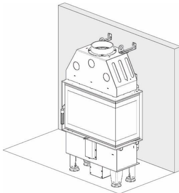
Rysunek 9. Mocowanie do ściany
