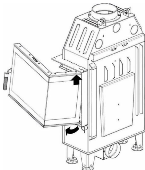
Krok 3. Podnieść drzwi maksymalnie w górę, aby wyjąć dolny trzpień zawiasu z tulei na dole ramy. Przechylić od dołu drzwi → na zewnątrz, aby dolny trzpień zawiasu znalazł się poza ramą.
