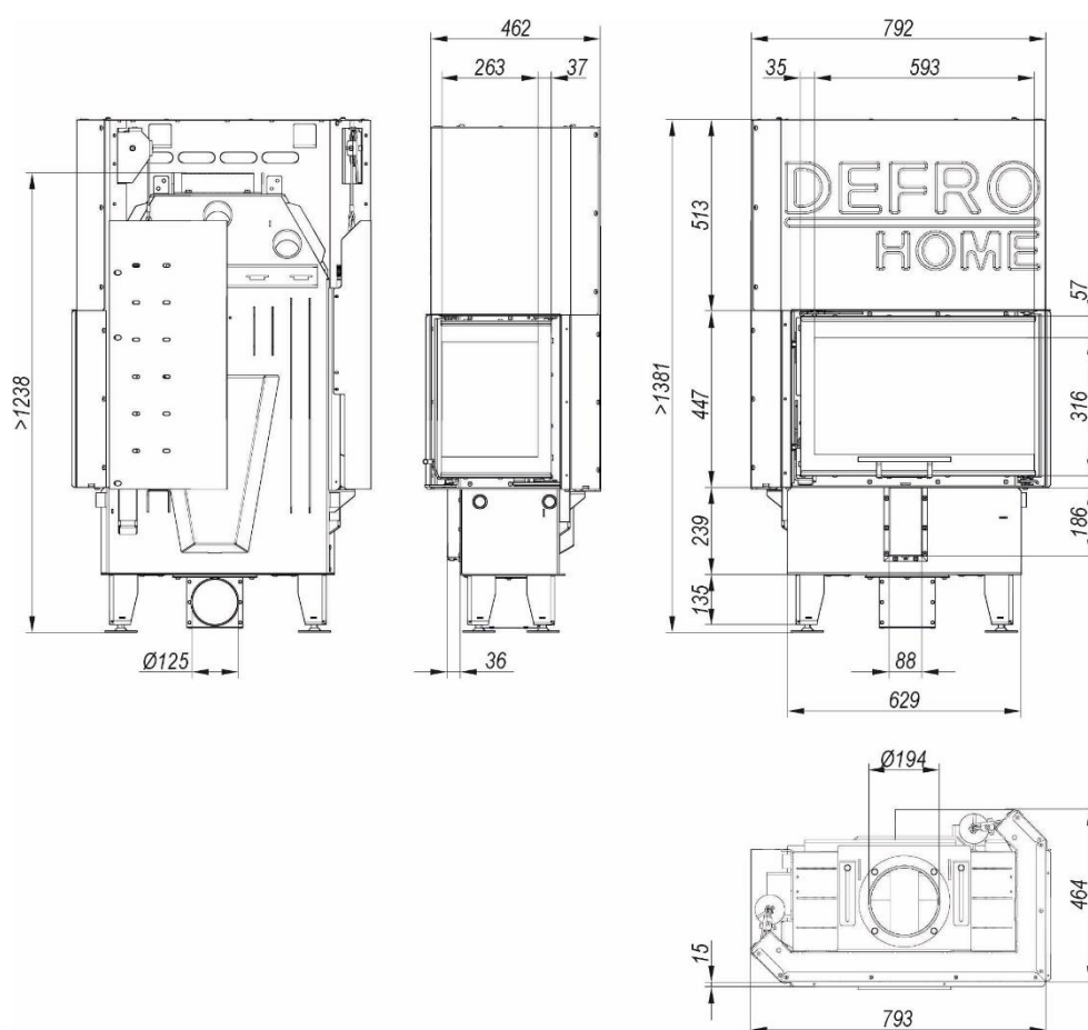
Rysunek 8. Wymiary wkładu kominkowego DEFRO HOME INTRA S BP G SLIM.
