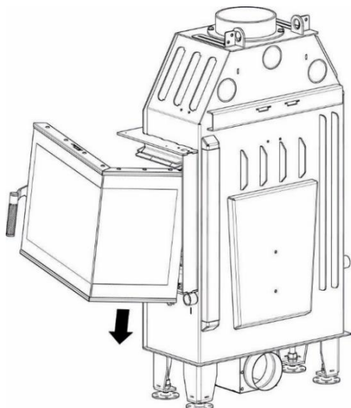
Rysunek 19. Sposób demontażu drzwi wkładu kominkowego
