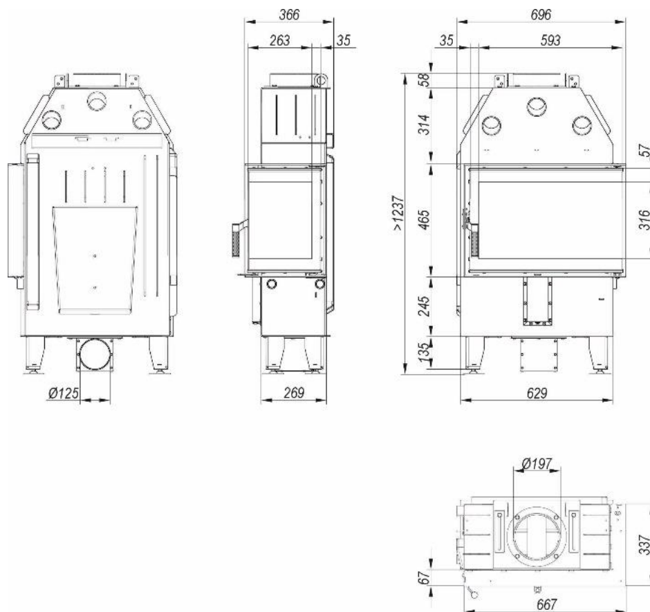
Rysunek 7. Wymiary wkładu kominkowego DEFRO HOME INTRA S BP SLIM.
