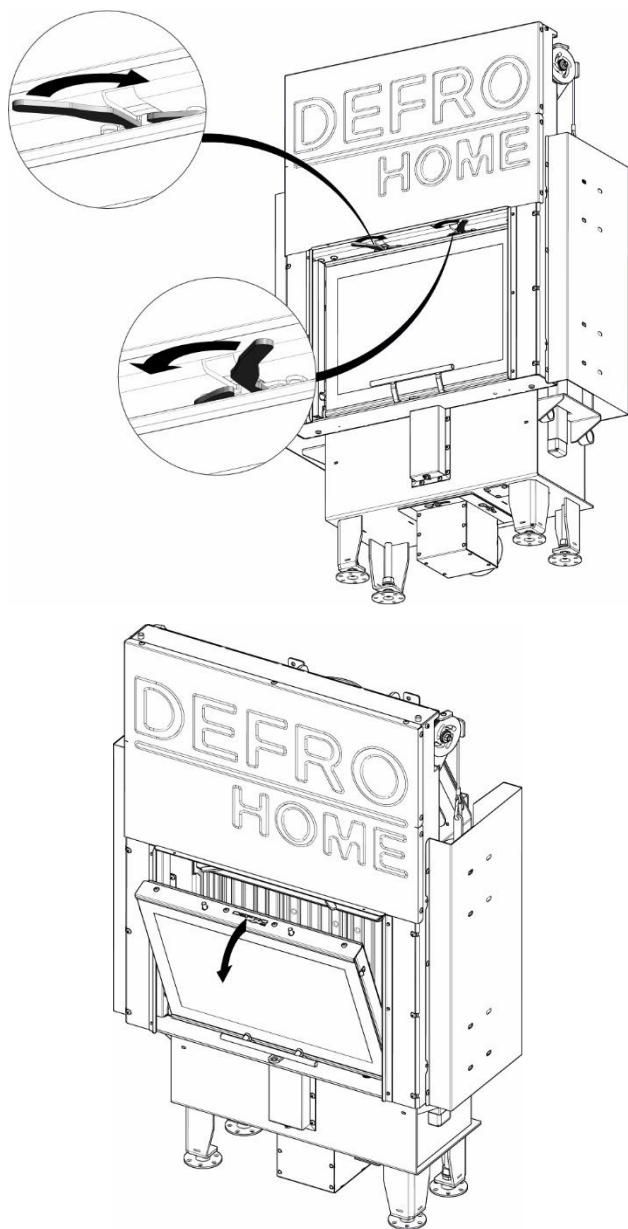
Rysunek 17. Umieszczenie rygli umożliwiających uchylne otwarcie drzwi gilotynowych wkładu kominkowego DEFRO HOME INTRA G SLIM.
