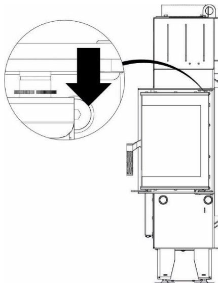
Krok 1. Zsunąć pierścień zabezpieczający maksymalnie w dół
