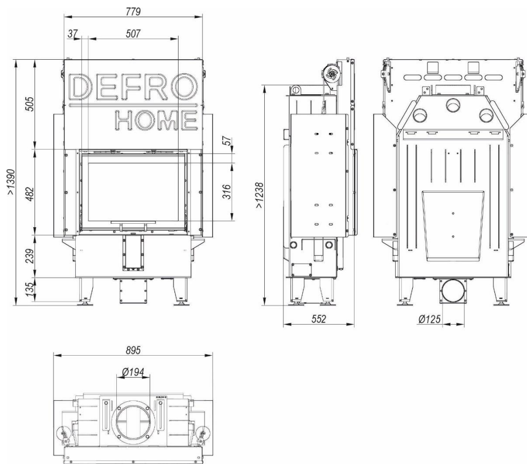
Rysunek 6. Wymiary wkładu kominkowego DEFRO HOME INTRA S G SLIM.
