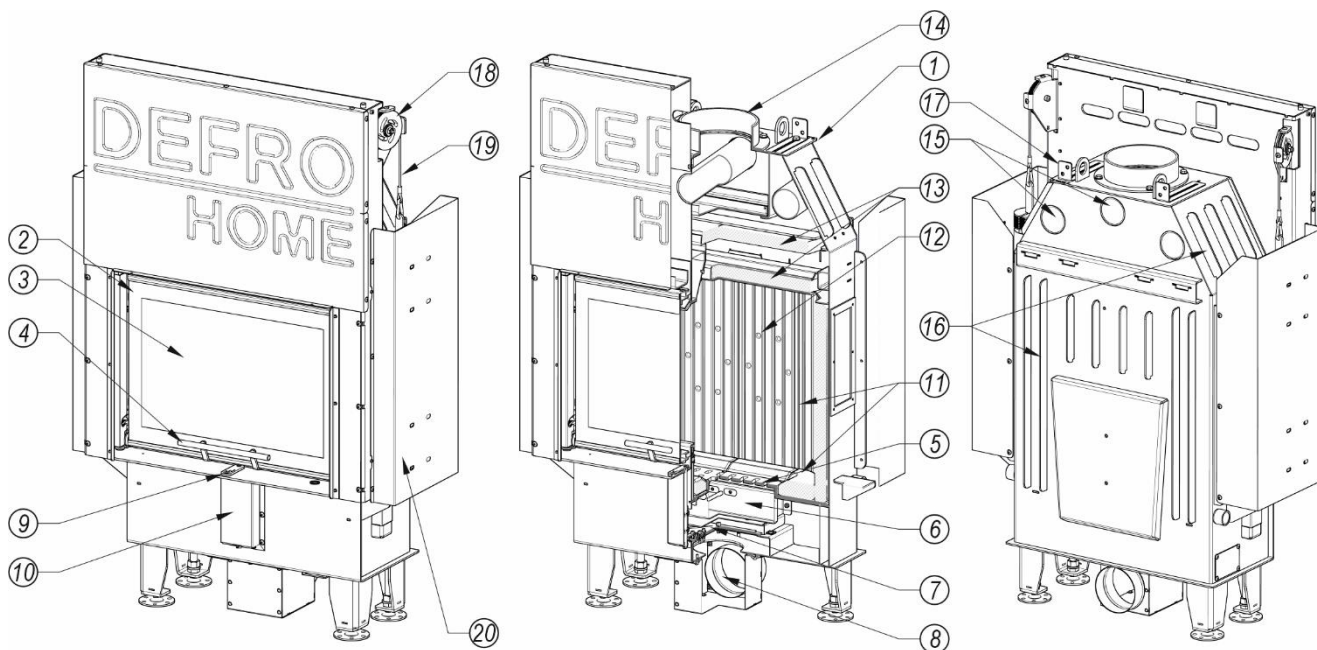
Rysunek 2. Budowa wkładu kominkowego DEFRO HOME INTRA S G SLIM
