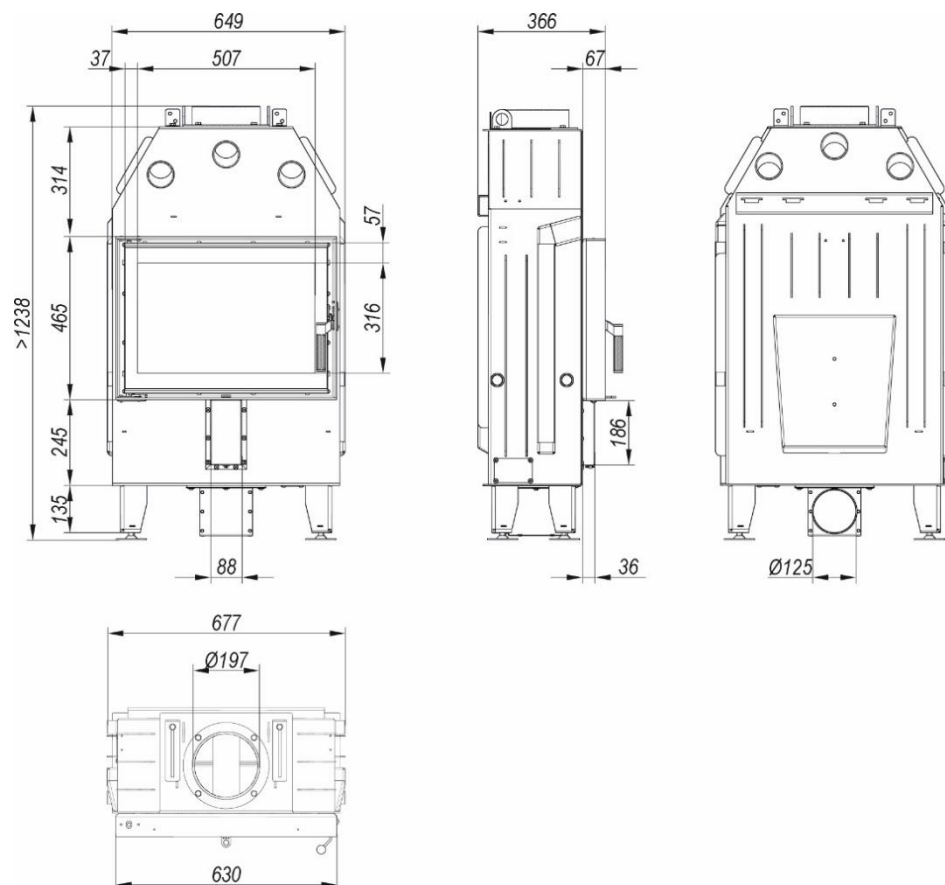
Rysunek 5. Wymiary wkładu kominkowego DEFRO HOME INTRA S SLIM.
