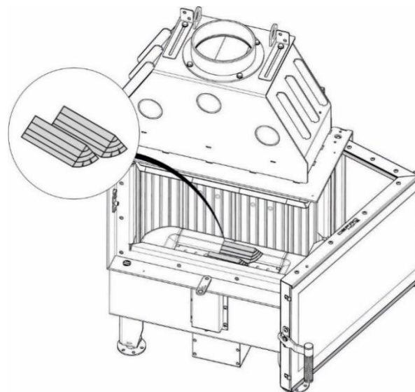
Rysunek 15. Sposób ułożenia paliwa
