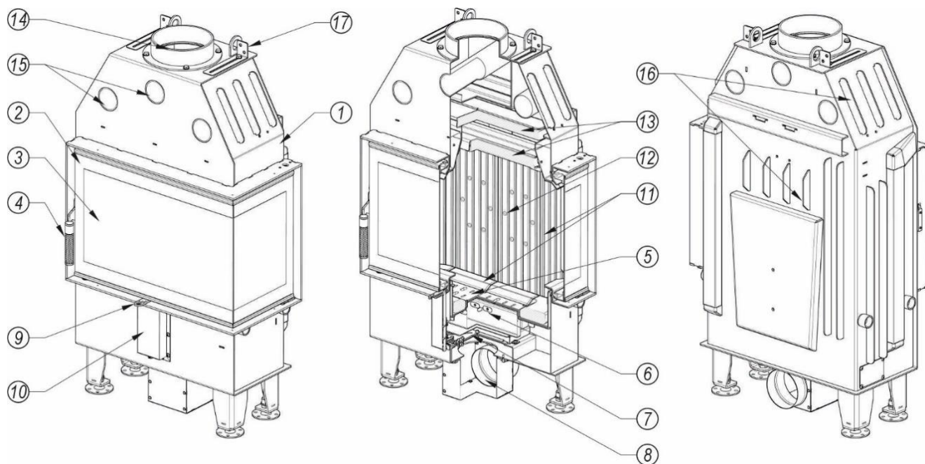
Rysunek 3. Budowa wkładu kominkowego DEFRO HOME INTRA S BP SLIM
