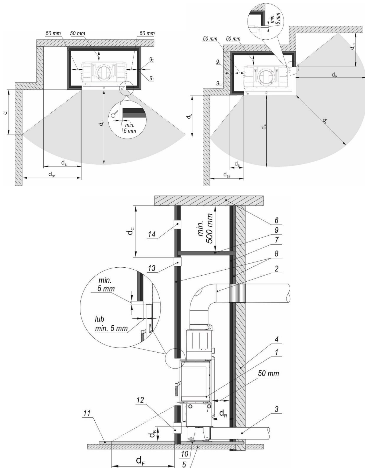
Rysunek 10. Przykładowa zabudowa wkładu kominkowego
