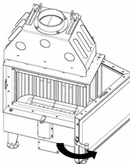
Krok 2. Otworzyć drzwi.
