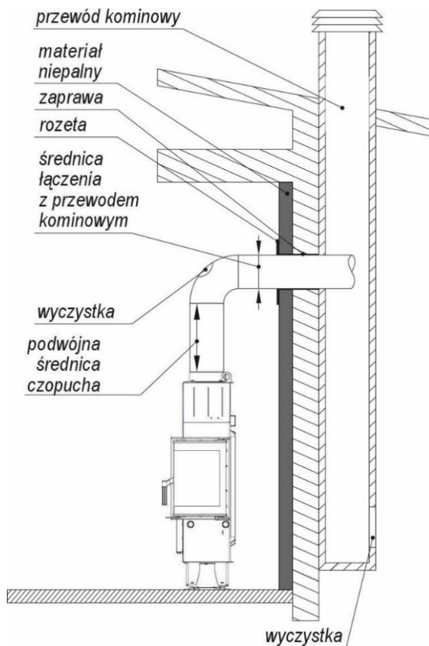
Rysunek 12. Podłączenie wkładu kominkowego do przewodu kominowego.
