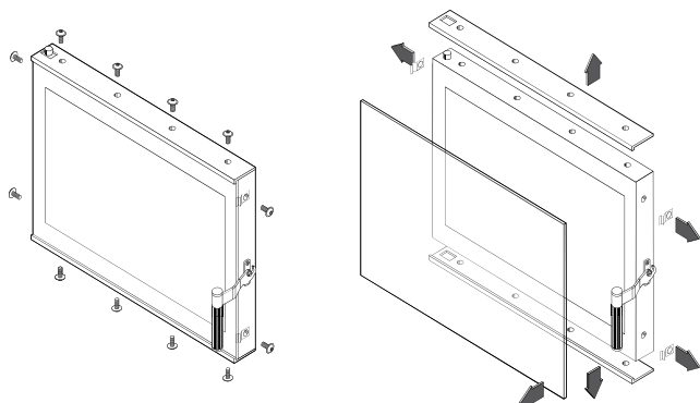
Rysunek 20. Demontaż szyby w drzwiach.
