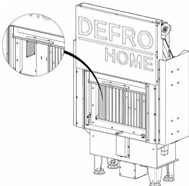
Rysunek 23. Umieszczenie pokryw otworów rewizyjnych we wkładach: DEFRO HOME INTRA SLIM wersji G
