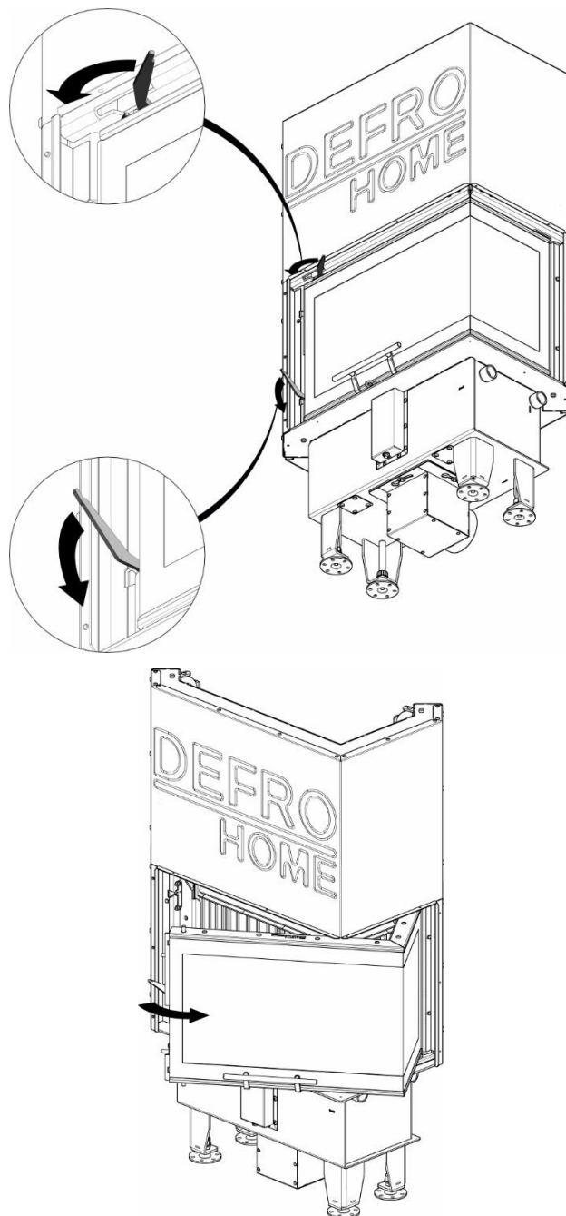
Rysunek 18. Umieszczenie rygli umożliwiających uchylne otwarcie drzwi gilotynowych wkładu kominkowego DEFRO HOME INTRA BP G SLIM.
