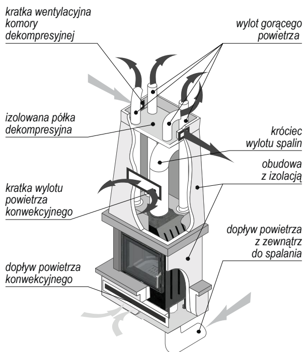
Rysunek 13. System dystrybucji gorącego powietrza.
