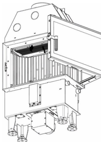
Rysunek 21. Sposób demontażu deflektora
