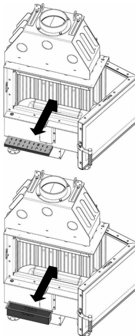
Rysunek 16. Wyjęcie rusztu i popielnika w celu jego opróżnienia.
