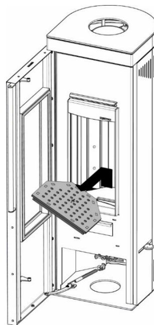
Rysunek 8. Ruszt ogrzewacza
