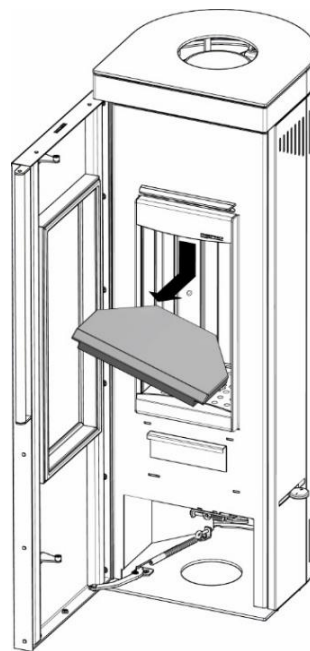
Krok 1. Jako pierwszy element należy zdemonstrować deflektor.
