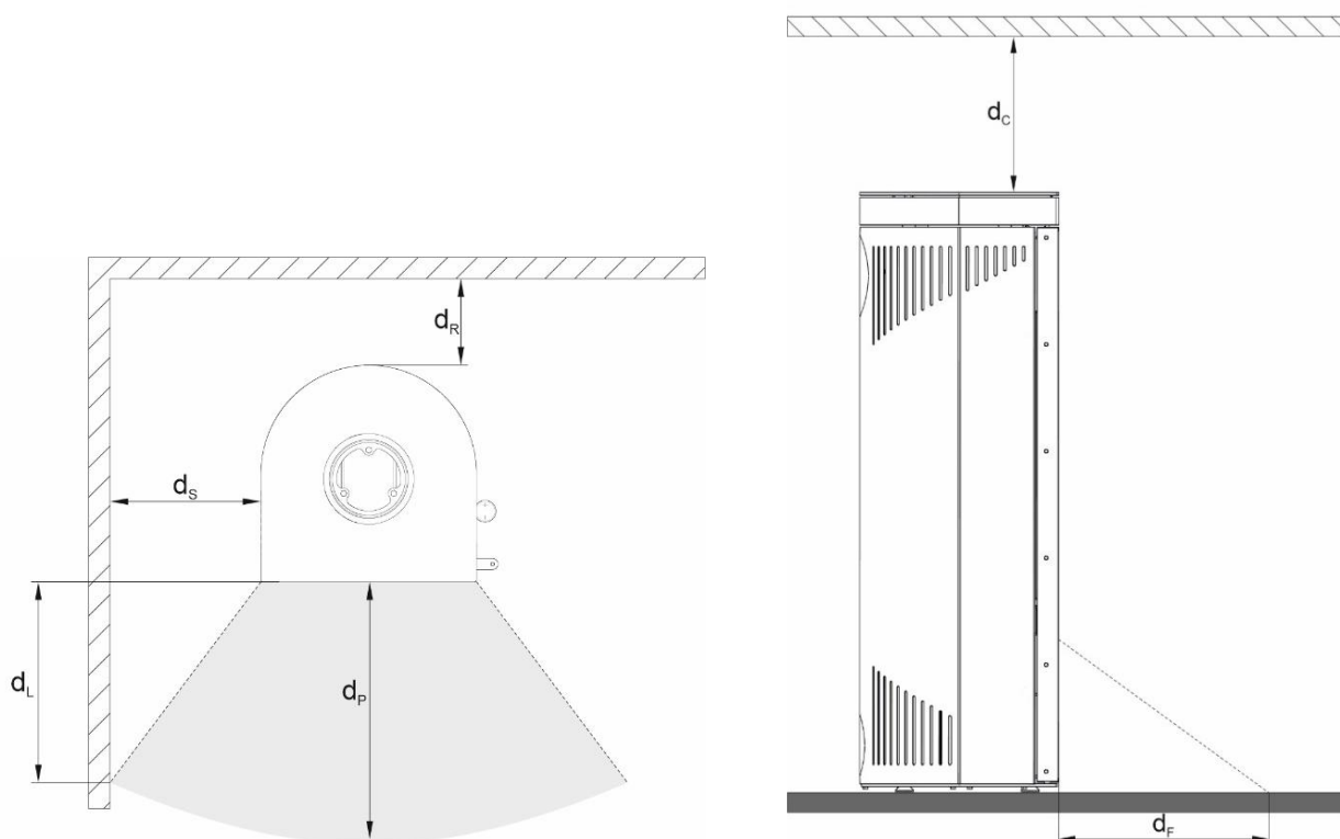
Rysunek 3. Odległości do materiałów palnych
