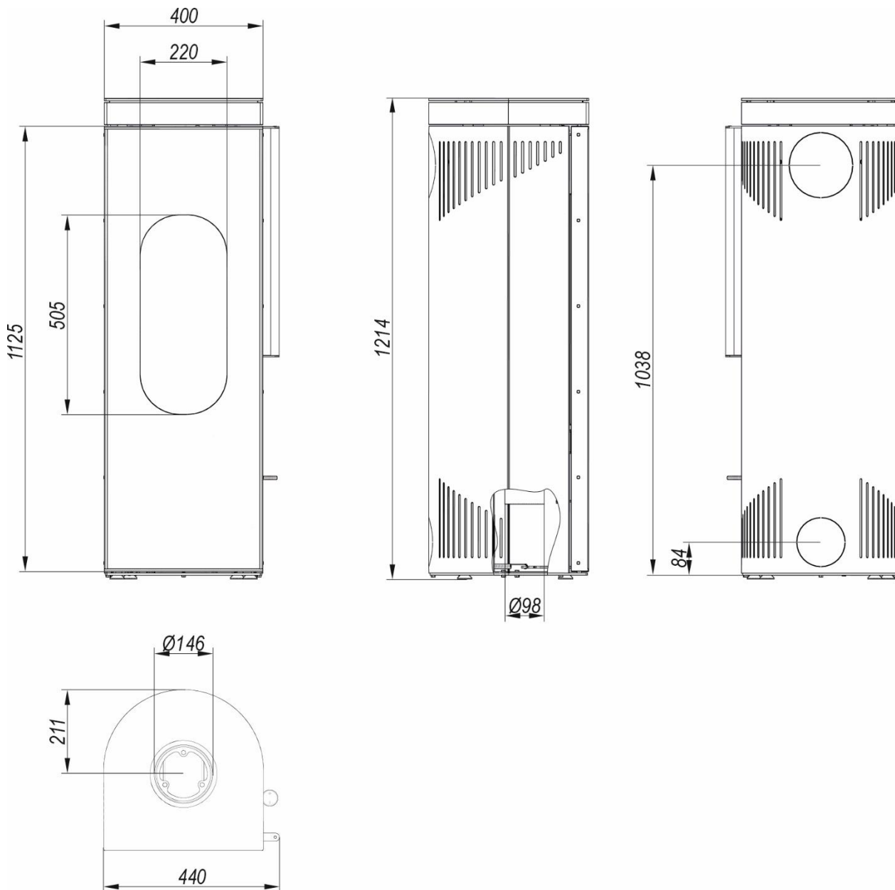
Rysunek 2. Wymiary ogrzewacza DEFRO HOME SOLIS
