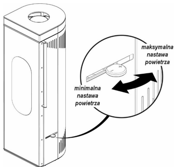
Rysunek 6. Ustawienie suwaka regulacji dopływu powietrza.
