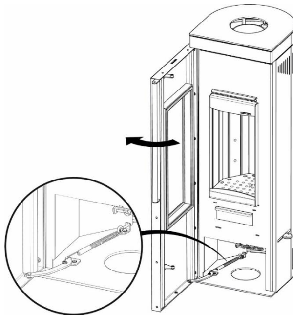
Rysunek 10. Mechanizm samodomyku drzwi
