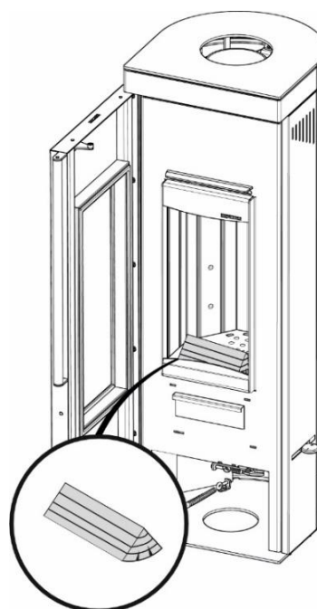
Rysunek 7. Sposób ułożenia paliwa.
