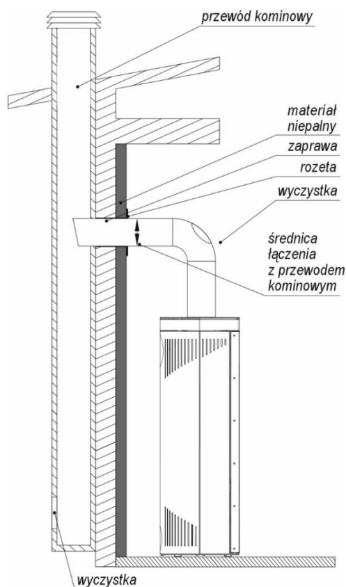
Rysunek 5. Podłączenie ogrzewacza do przewodu kominowego.
