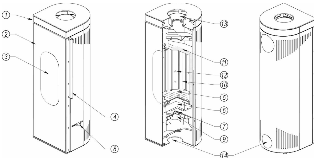
Rysunek 1. Budowa ogrzewacza pokojowego DEFRO HOME SOLIS
